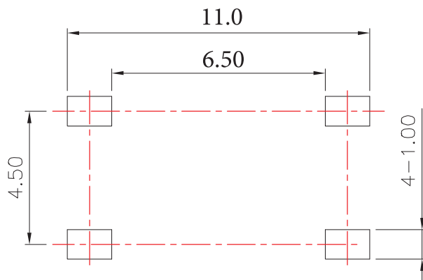
PCB Lavout(Pattern side)
