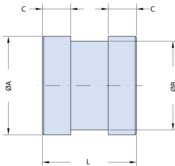
10-101033-13 10-305045-XX
