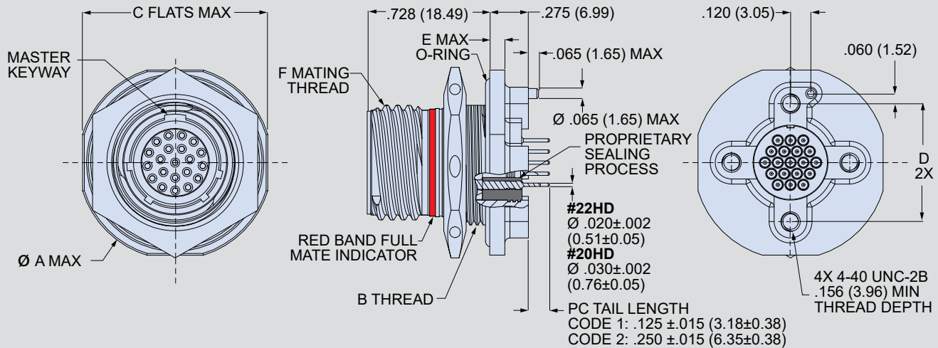
806-028 Receptacle Dimensions
