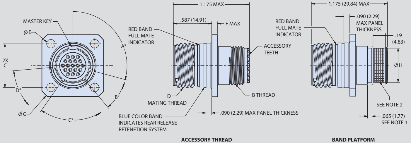
806-052 Receptacle Dimensions
