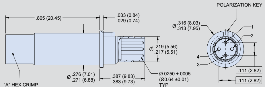
Pin Contact 854-047
