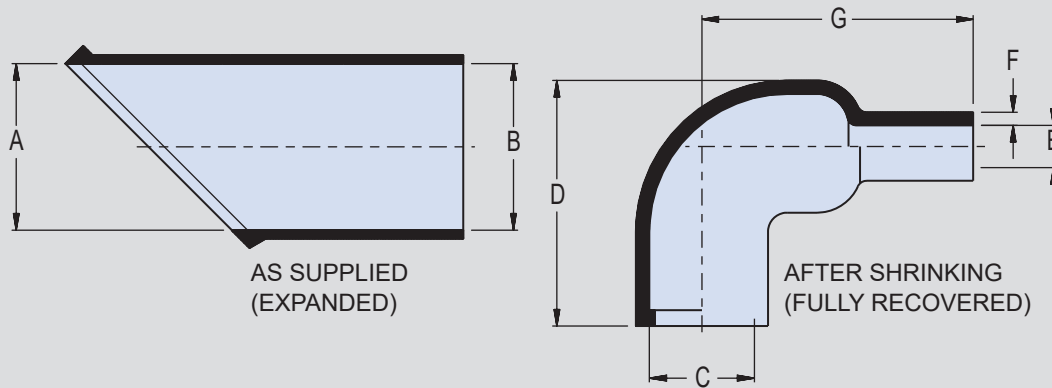
809A060 90° Boots
