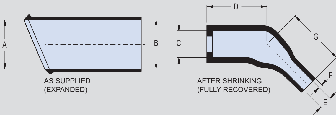
809B060 45° Boots
