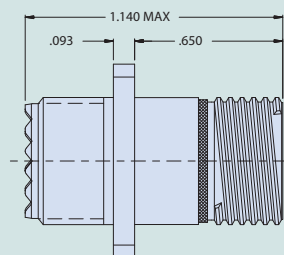
07- Wall Mount Receptacle
