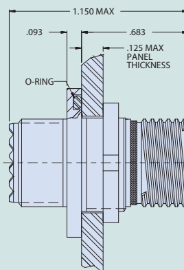
08- Jam Nut Receptacle
