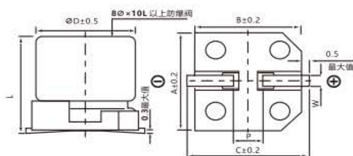
ΦD=4~10 适用
