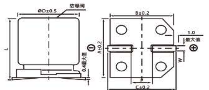
\varnothing 12.5 以上适用
