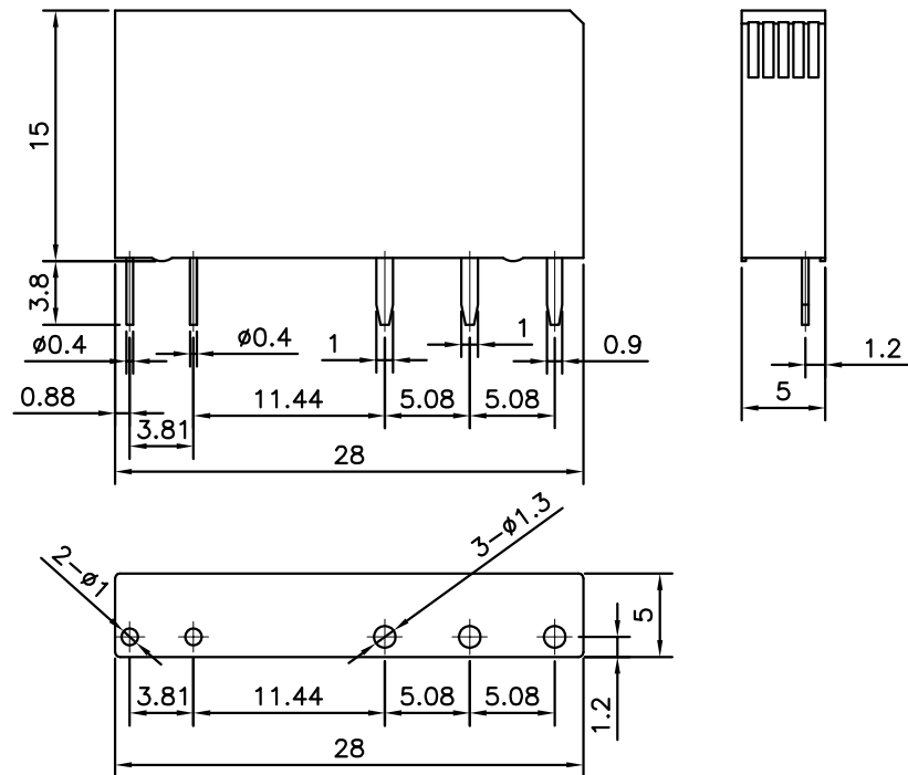
P.C.B LAYOUT
