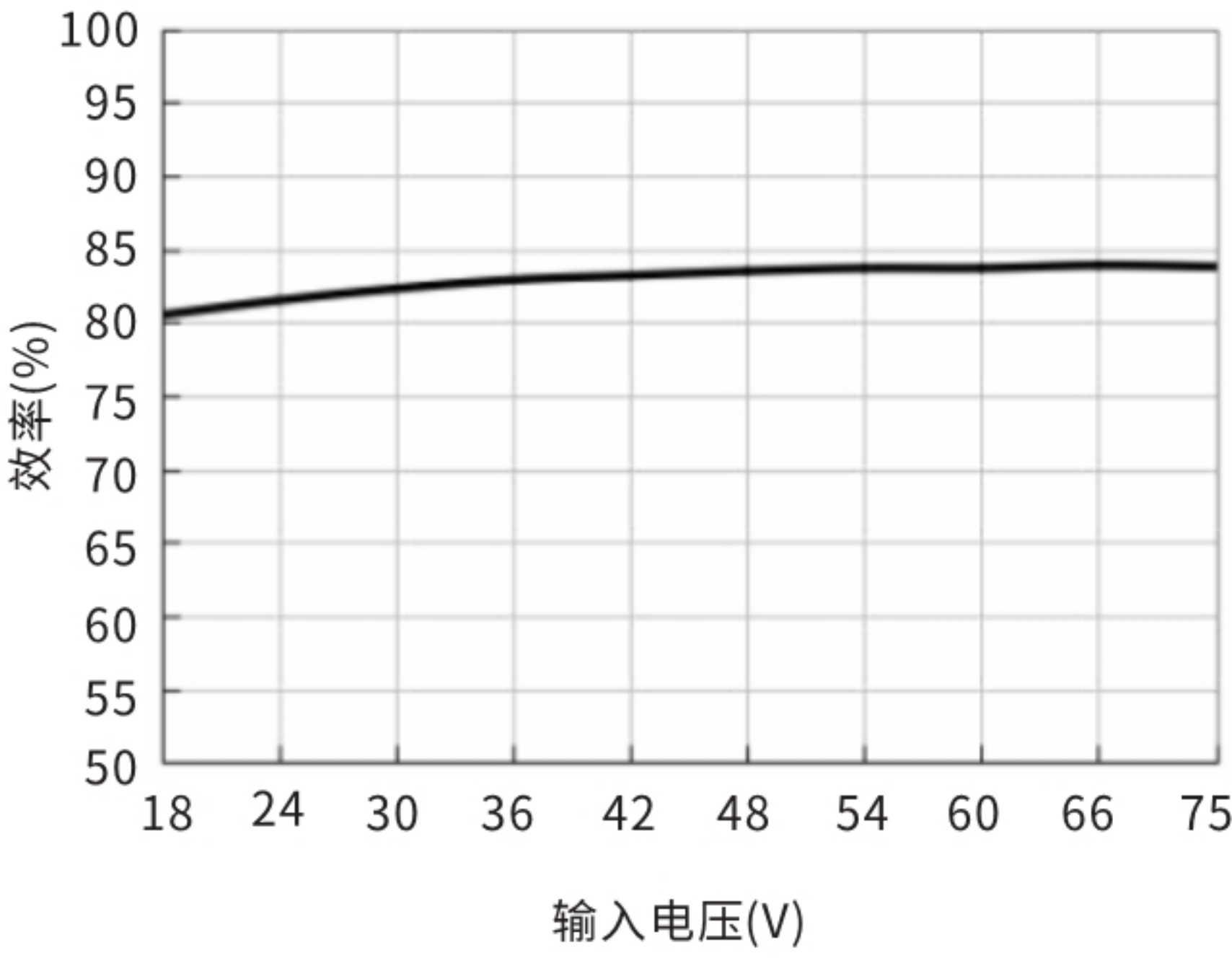
效率Vs输入电压(满载) URA4815YMD-6WR3
