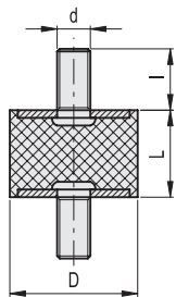
DVA.1-SST
