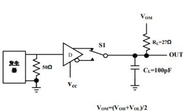
图 3 驱动器差分延迟与渡越时间
