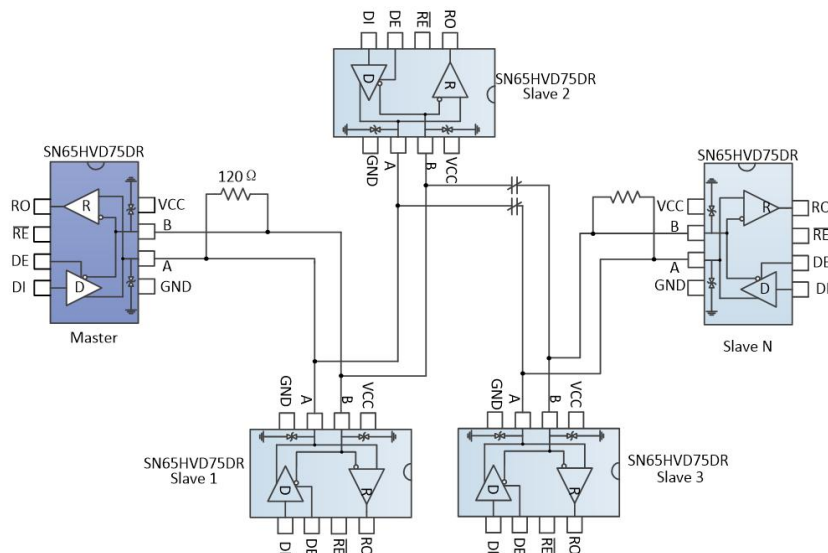
图 10 手拉手式 RS485 半双工通讯网络
