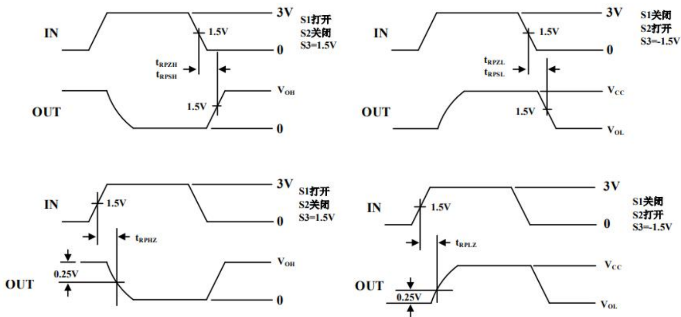
图 8 接收器使能与禁能时间
