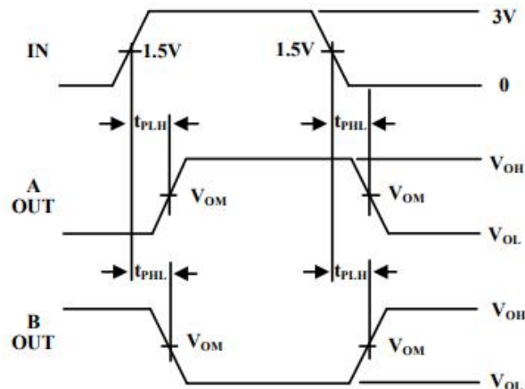
图 4 驱动器传播延迟
