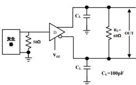
图 2 驱动器直流测试负载
