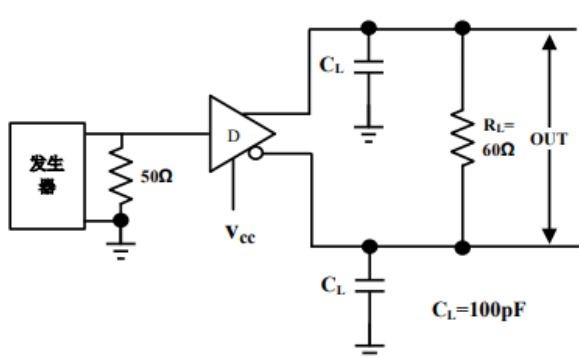
图 2 驱动器直流测试负载
