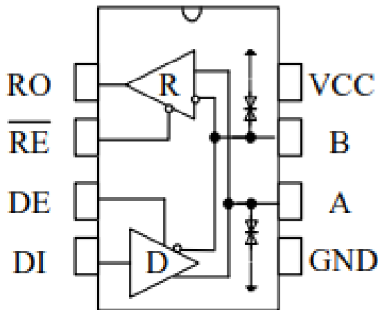
图 1 ESGM3085E 引脚分布图
