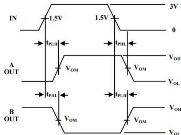
图 4 驱动器传播延迟
