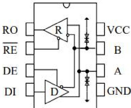
图 1 ES3088E 引脚分布图
