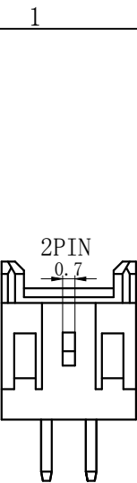
2PIN
