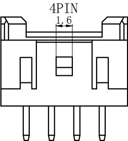
4PIN
