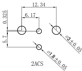
PCB 安装尺寸
