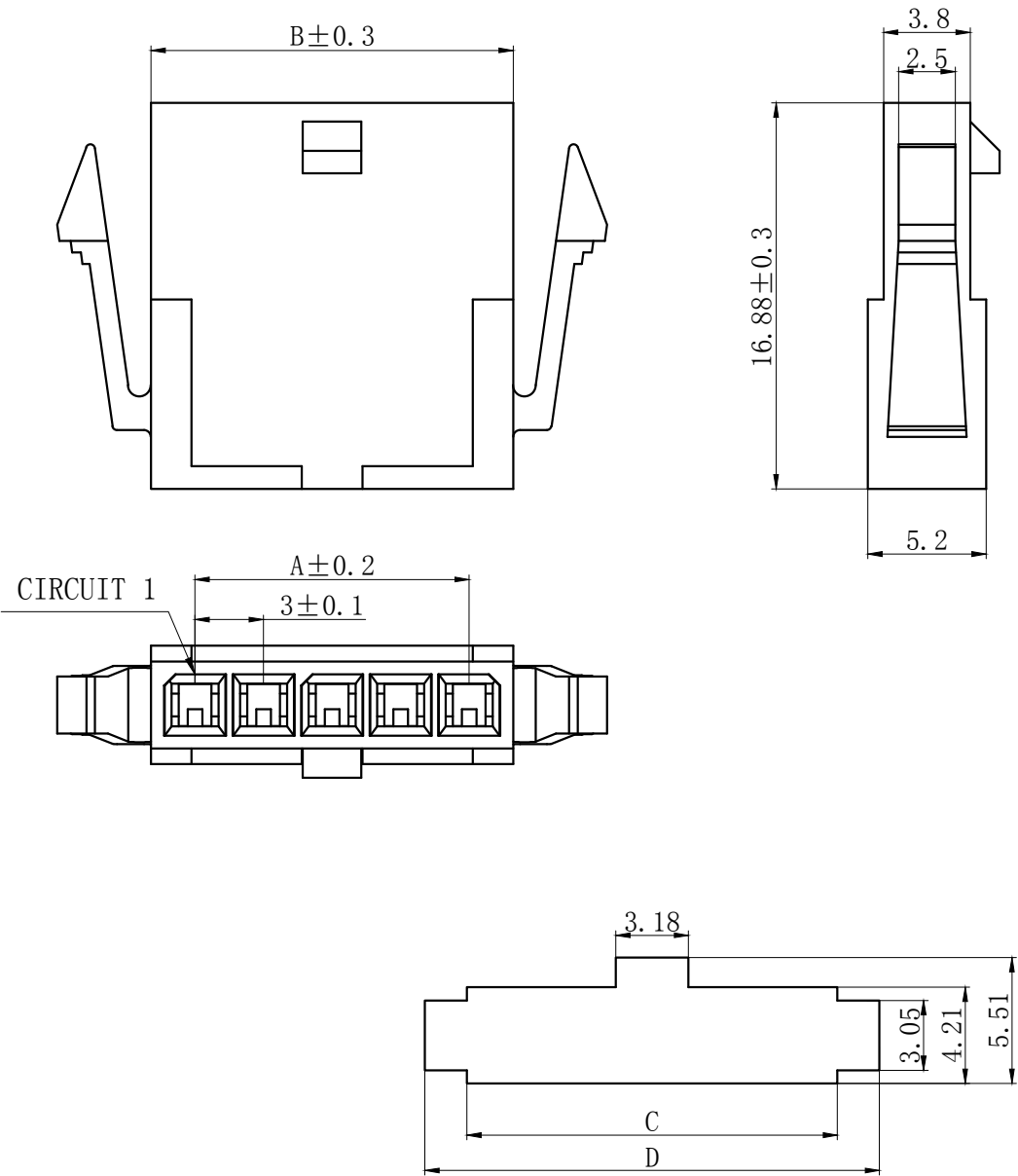
安装尺寸
