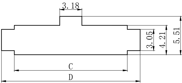
安装尺寸
