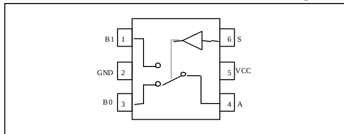
SC70
