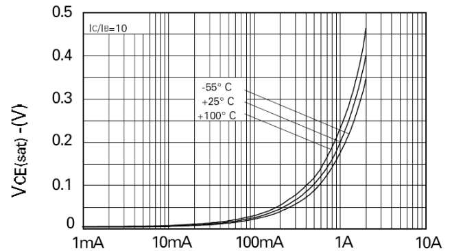
V_{CE(sat)} \text{ v } I_C
