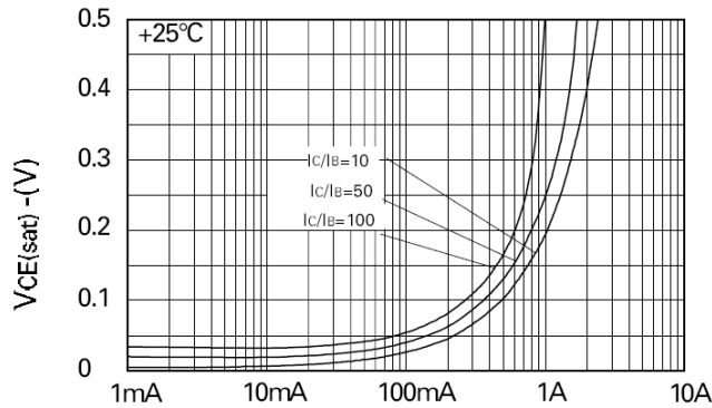
V_{CE(sat)} \text{ v } I_C
