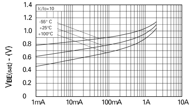
V_{BE(sat)} \text{ v } I_C
