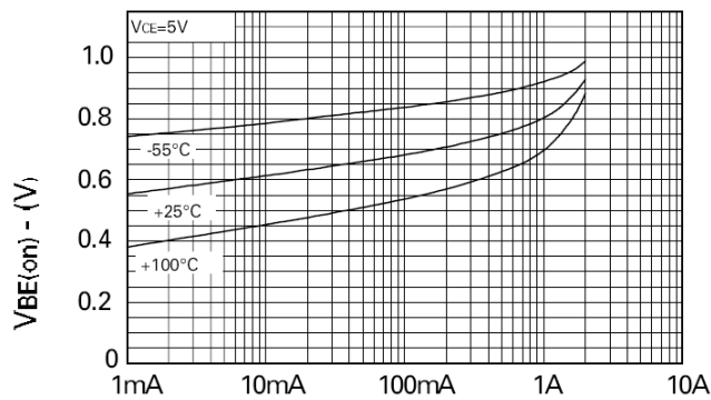
V_{BE(on)} \text{ v } I_C
