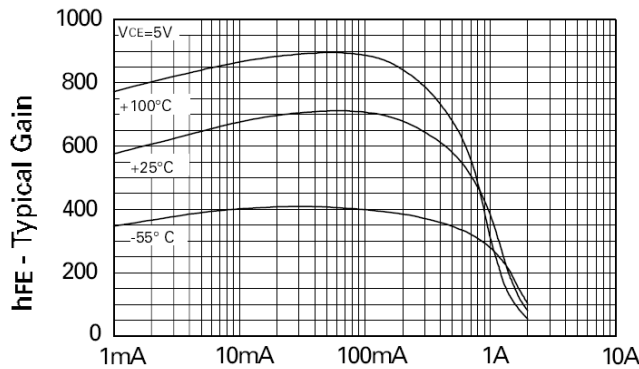
h_{FE} \text{ v } I_C
