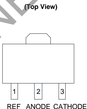
SOT-89 (Option 1)
