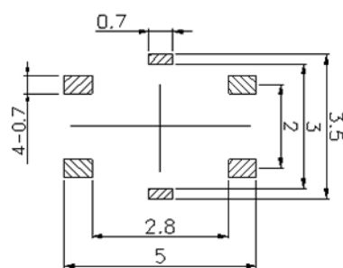
PCB. 焊接图
