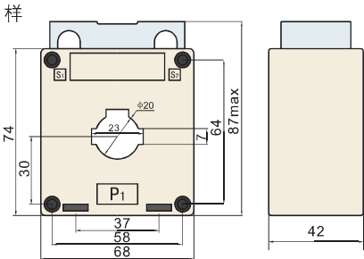
LMK-0.66 20型图
