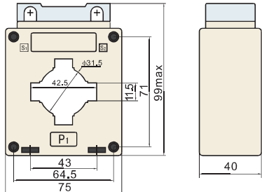
LMK-0.66 40型图样
