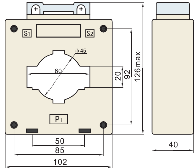
LMK-0.66 60型图样
