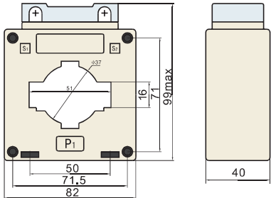
LMK-0.66 50型图样
