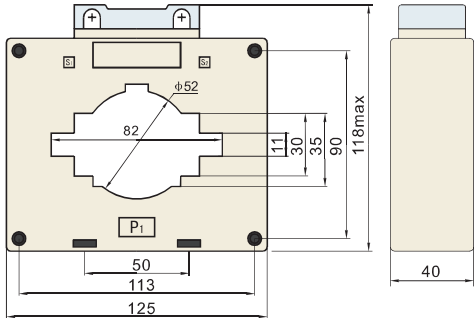
LMK-0.66 80型图样
