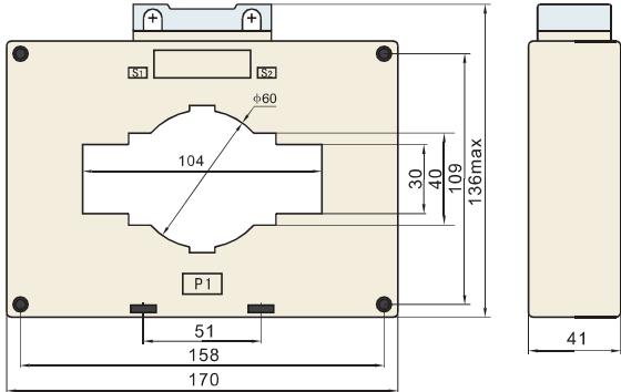
LMK-0.66 100型图样
