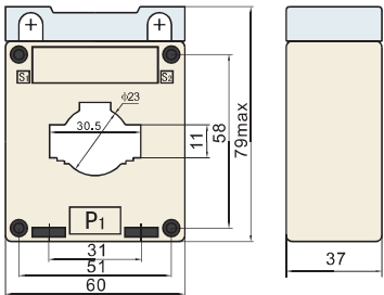
LMK-0.66 30型图样
