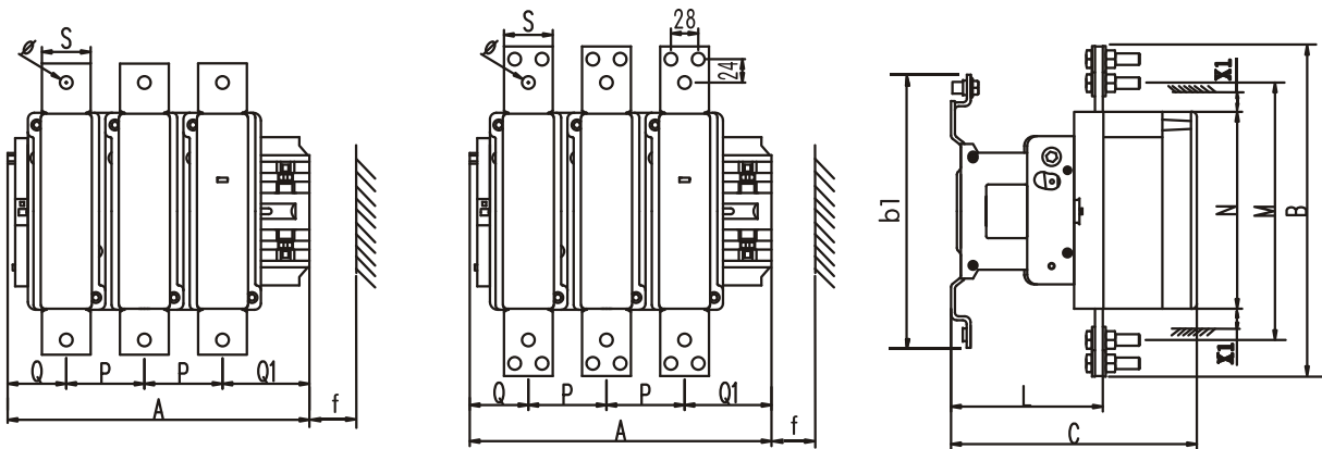
CJX2sF-1000、1250 外形
