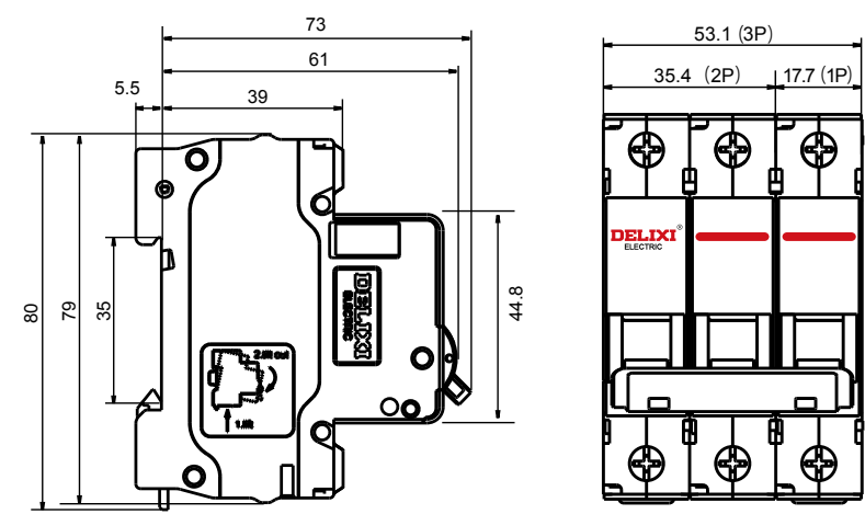
外形及安装尺寸（mm）
