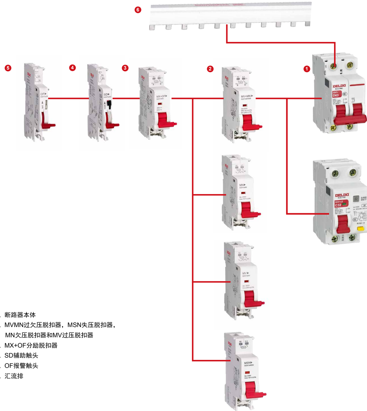
DZ47v 附件安装示意图
