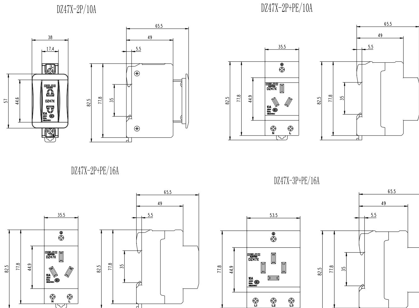
DZ47X 框缘式插座 (模数化插座)
