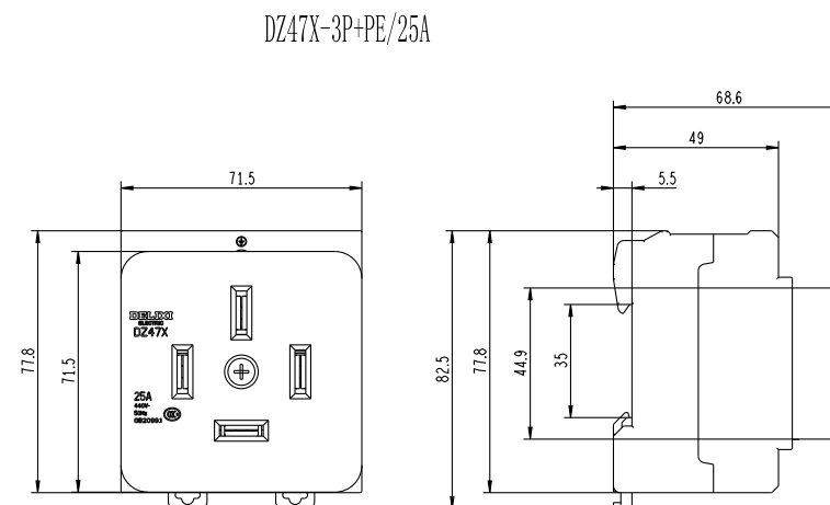
DZ47X 框缘式插座 (模数化插座)
