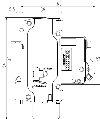
1P+N右视图
