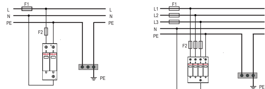
TT 系统安装示意图
