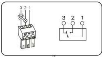
接线能力：1.5mm 2 (max) U max ：AC125V I max ：1A
