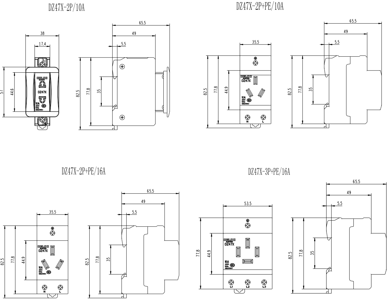
DZ47X 框缘式插座（模数化插座）
