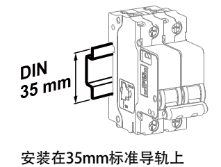
安装在35mm标准导轨上
