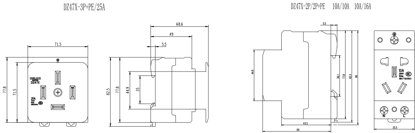
DZ47X 框缘式插座（模数化插座）
