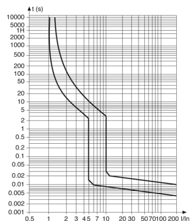
C 曲线
