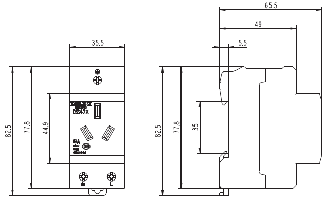
DZ47X-2P+PE/10A
