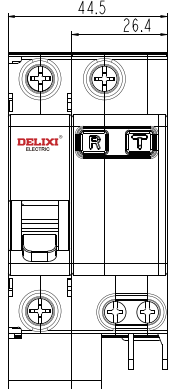
1P+N-32A
