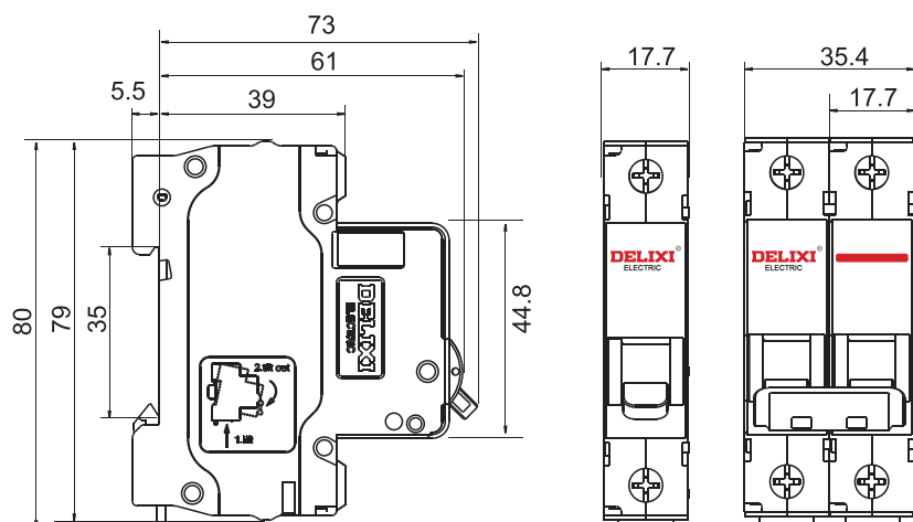
DZ47s-80 小型标准断路器
