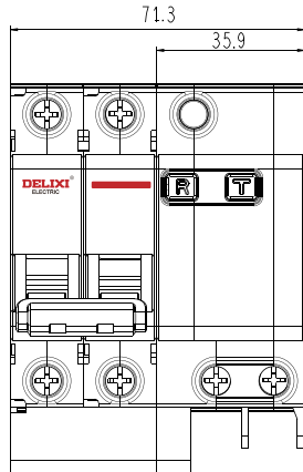
2P-63A
