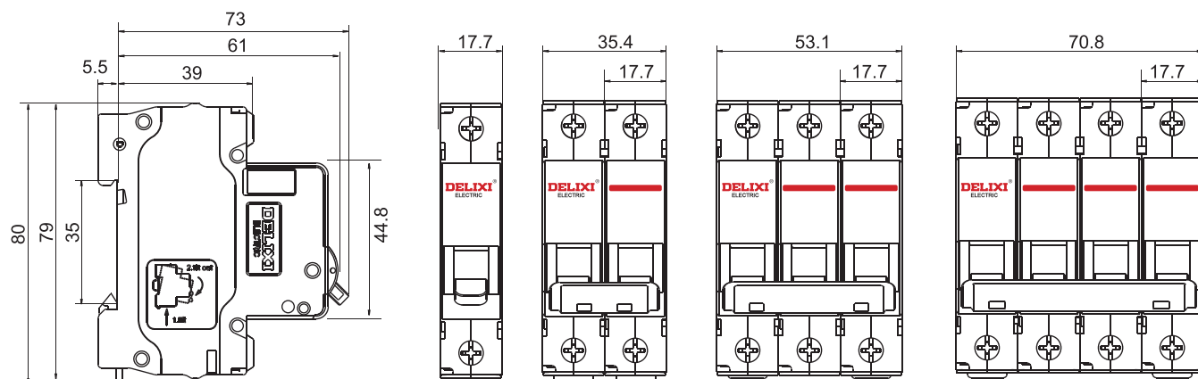
DZ47s 小型标准断路器
