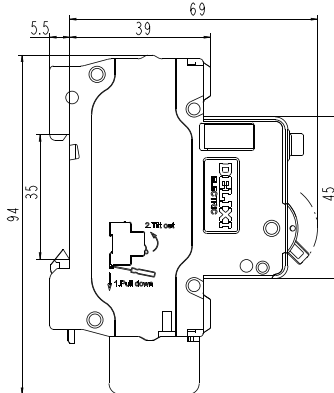
1P+N右视图
