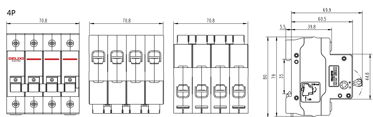
DZ47G 隔离开关
