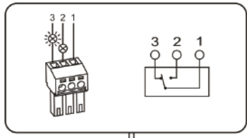
接线能力： 1.5mm^2(max) U_{max} : AC125V I_{max} : 1A
