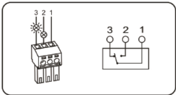
接线能力：1.5mm²(max) Umax: AC125V Imax: 1A
