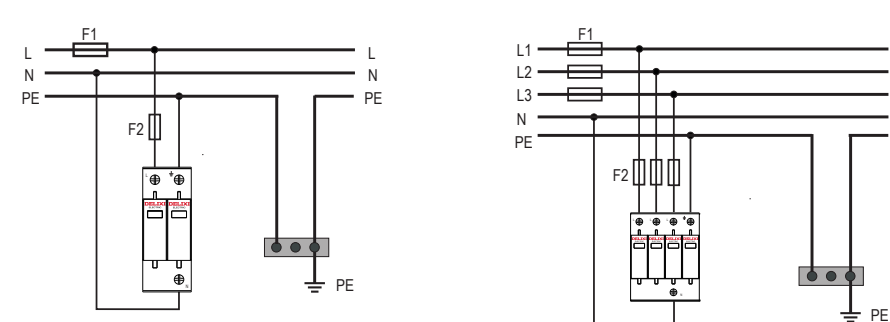
TT 系统安装示意图
