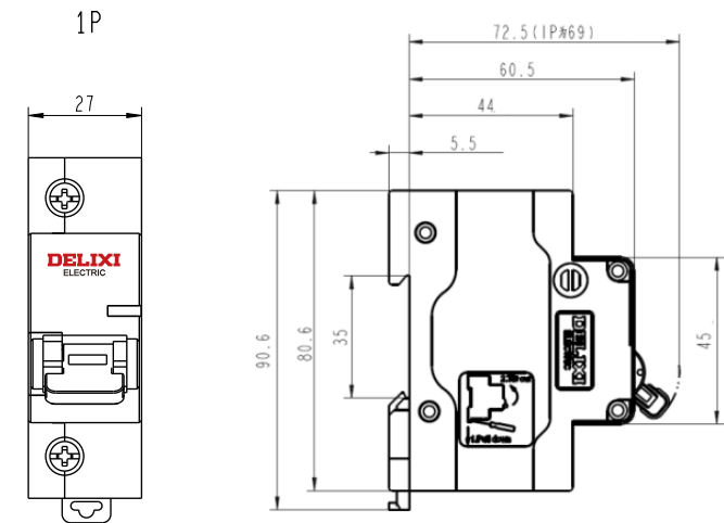
DZ47-125 大电流断路器
