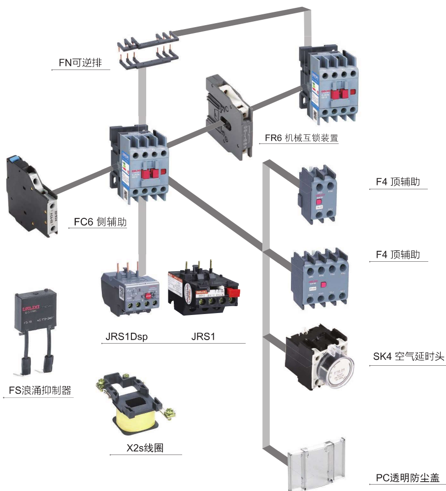
■ CJX2s-6-95A附件装备位置示意图
