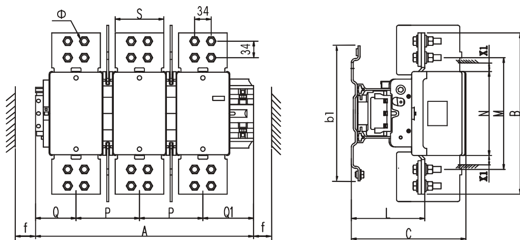
CJX2sF-1450、1700、2100 外形
