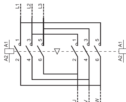
■ CJX2sF-115N~800N(水平安装, 机械互锁)
