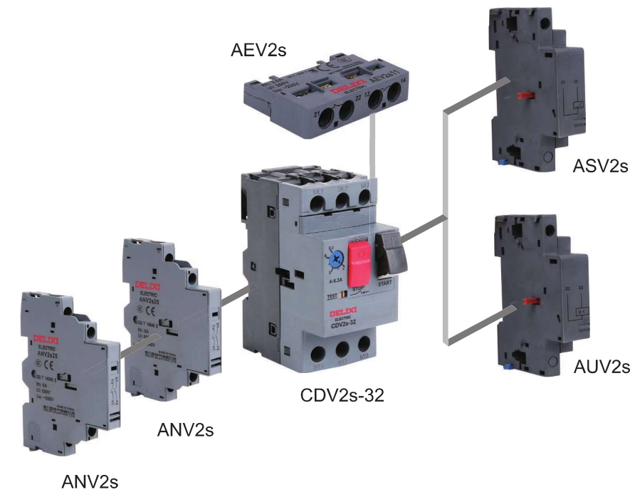
附件安装示意图
