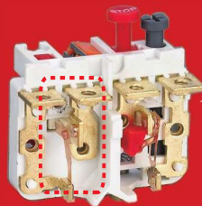
片簧式动触头
