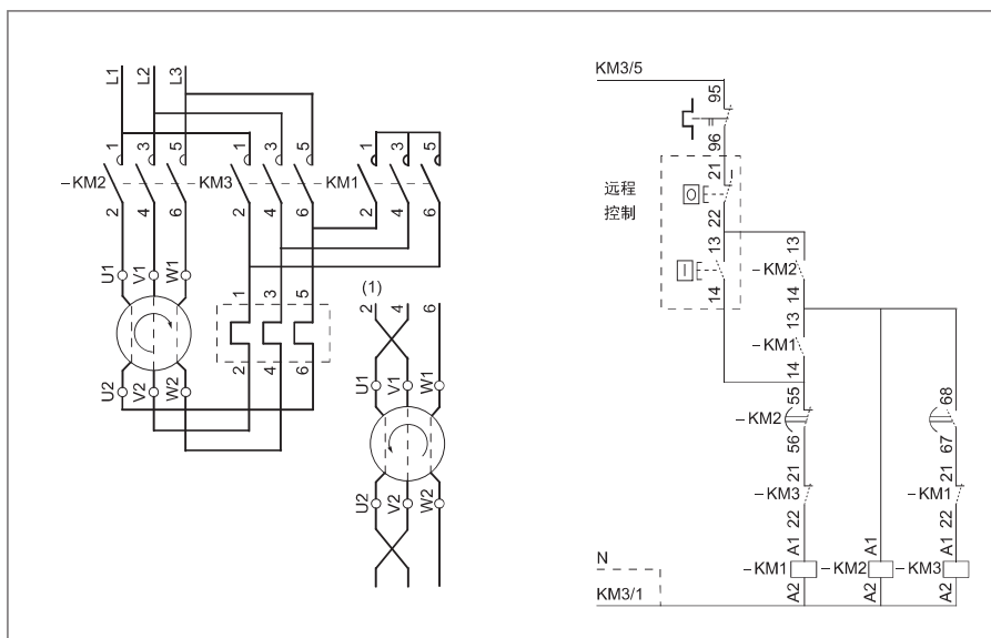
■ 星-三角起动器接线图
