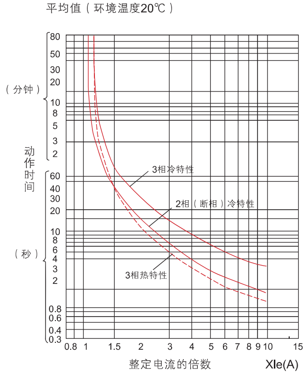
脱扣曲线图
