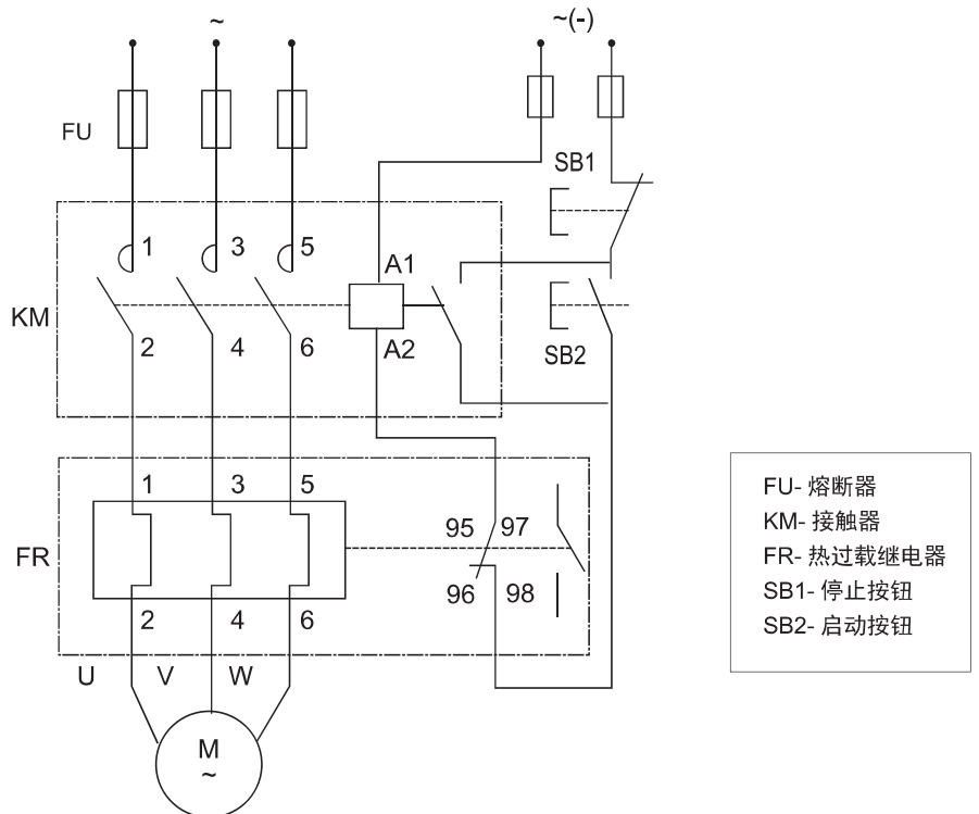
安装接线示意图
