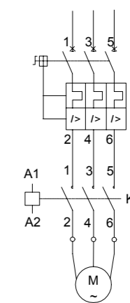
CDV2s配合CJX2s拖带负载
