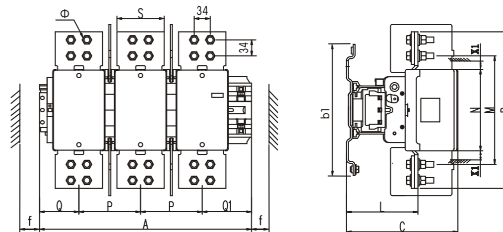
CJX2sF-1450、1700、2100 外形 CJX2sF-
