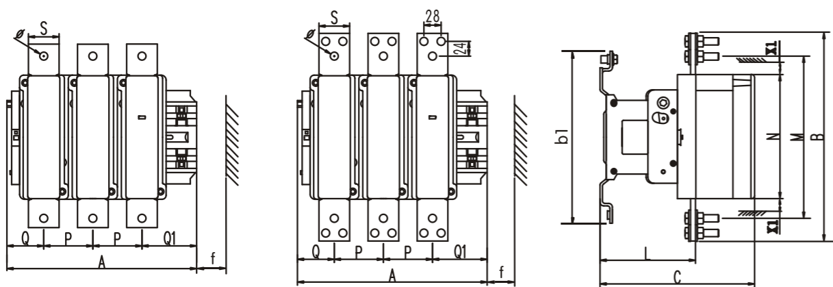
CJX2sF-1000、1250 外形
