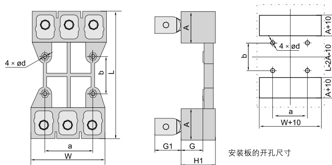
插入式板后的外形及安装尺寸
