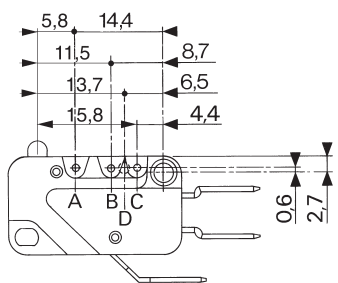
161E roller
