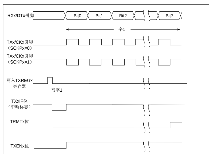
图 14-7: 同步发送 (通过 TXENx)
