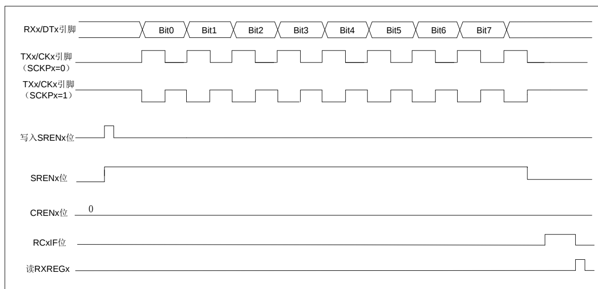
图 14-8：同步接收（主控模式，SREN）
