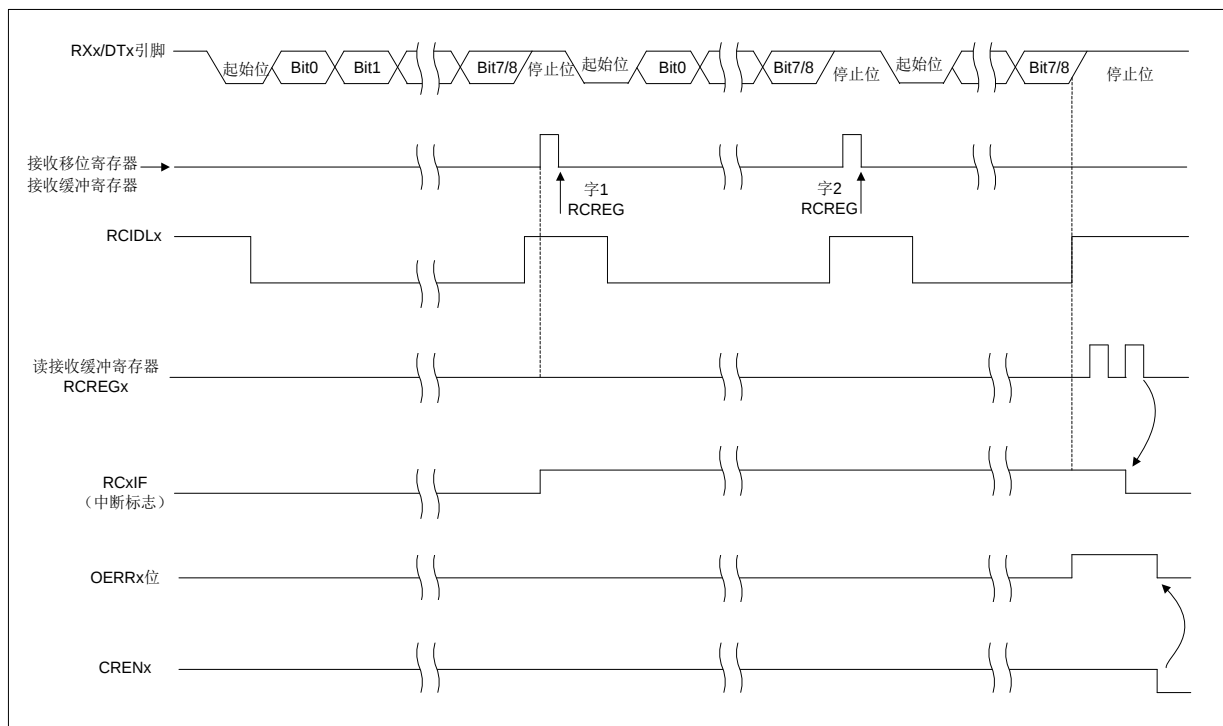
图 14-5: 异步接收
