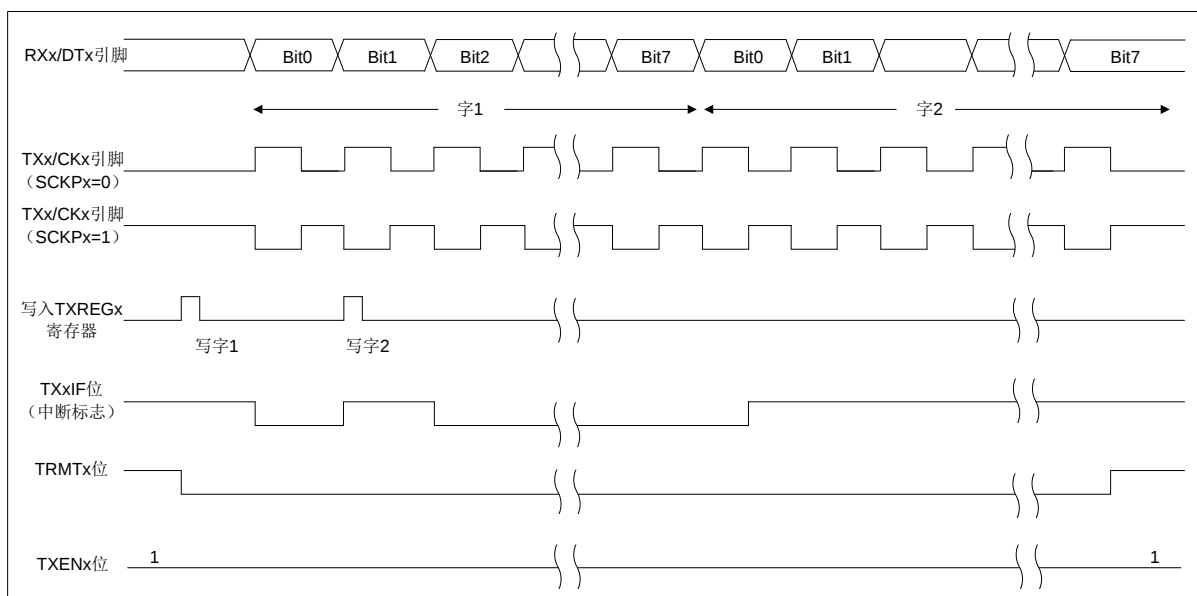
图 14-6: 同步发送
