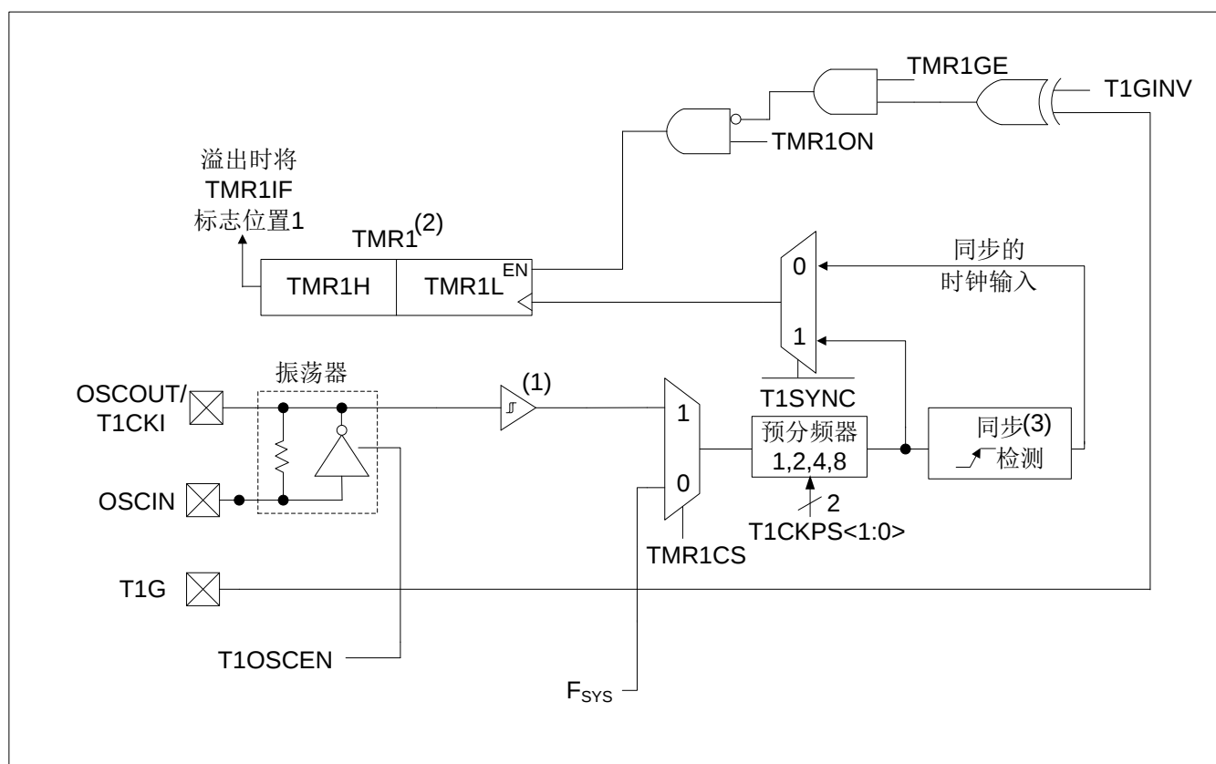
图9-1: TIMER1结构图
