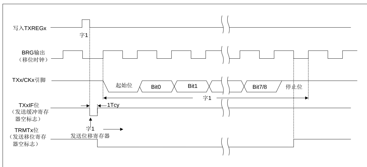
图 14-3: 异步发送
