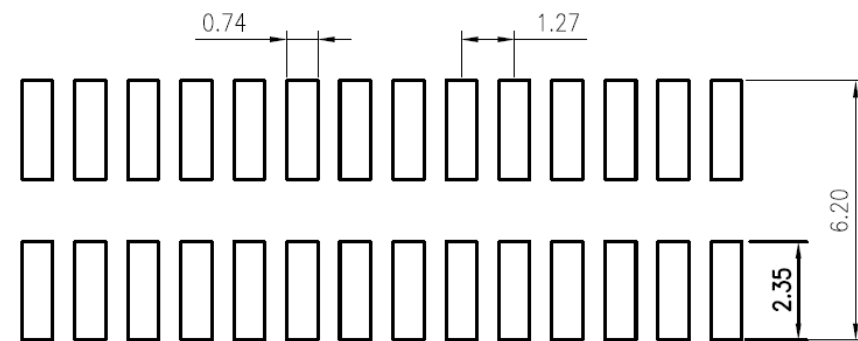
P.C.B LAYOUT
