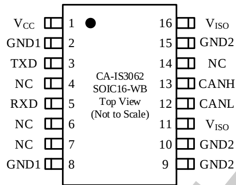
图 6-1 引脚配置
