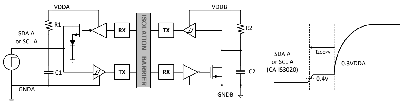
图 8-2. t_{\text{LOOPA}} 测试电路与波形
