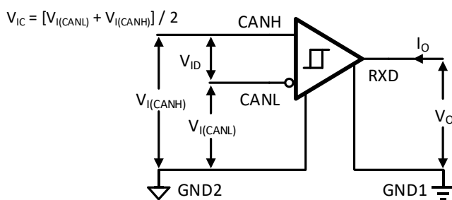
图 8-6 接收器输出电压、电流测试条件
