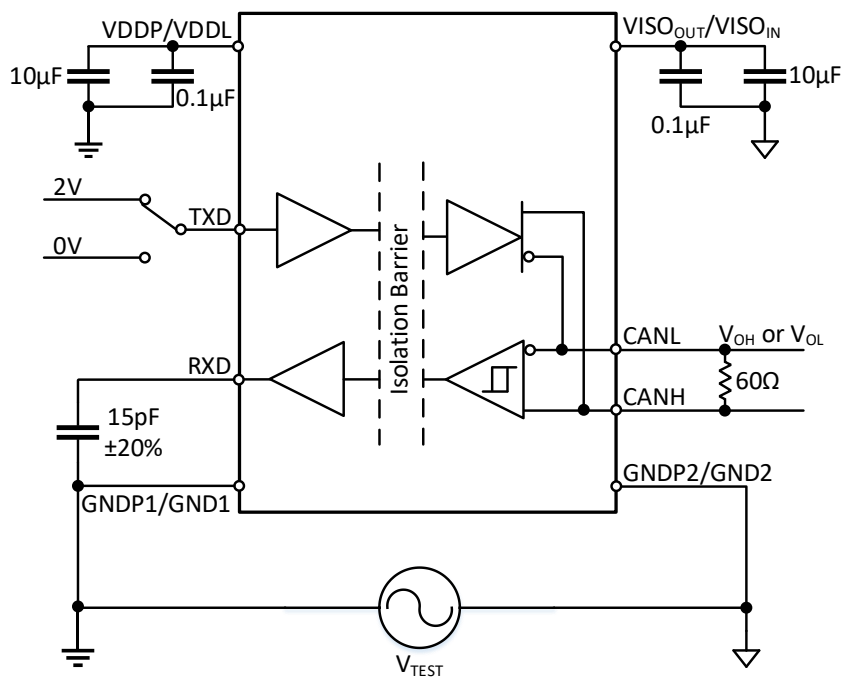
图 8-12 共模瞬态抑制比 (CMTI) 测试电路
