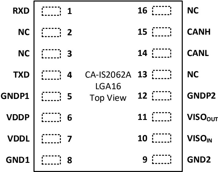
图 6-1 引脚分布图
