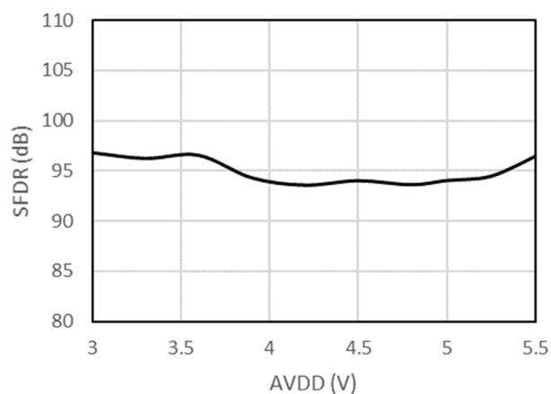
图 7-20 无杂散动态范围 vs 高边供电电压
