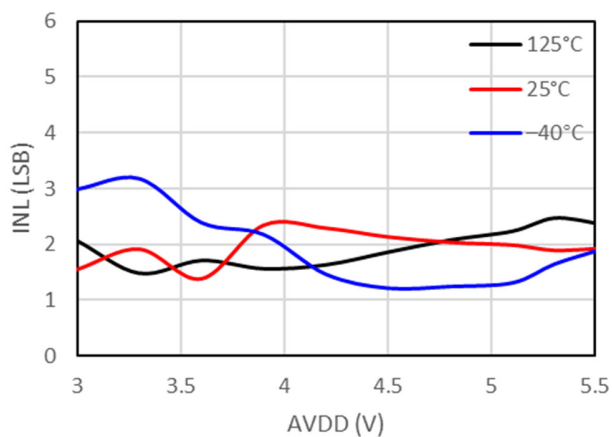
图 7-27 积分非线性 vs 高边供电电压
