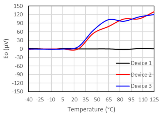
图 7-6 失调误差 vs 温度
