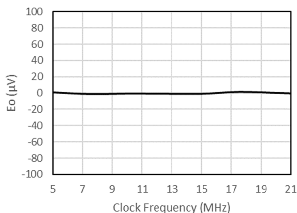
图 7-8 失调误差 vs 时钟频率
