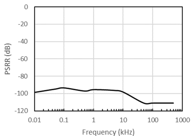
图 7-30 电源抑制比 vs 频率
