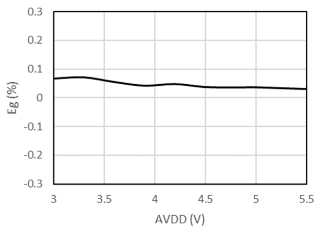
图 7-4 增益误差 vs 高边供电电压
