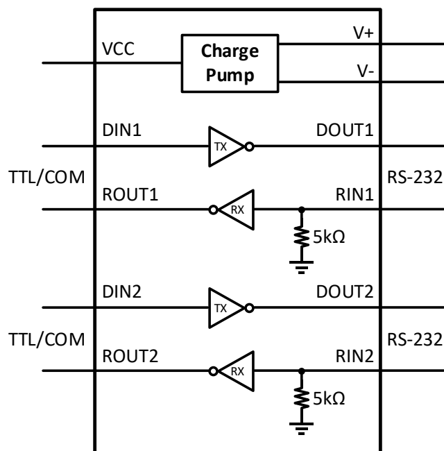
简化原理图
