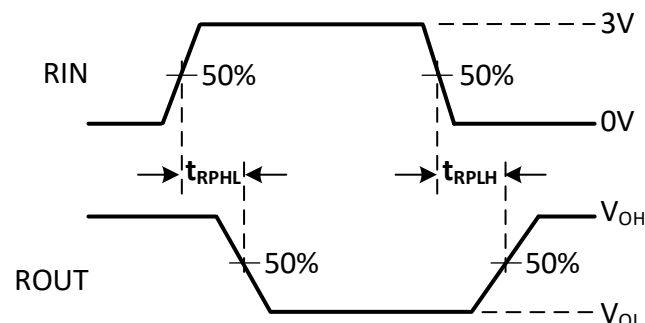
图 8-3 接收器传播延迟时间
