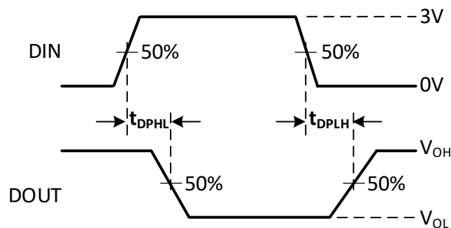
图 8-1 驱动器传播延迟时间
