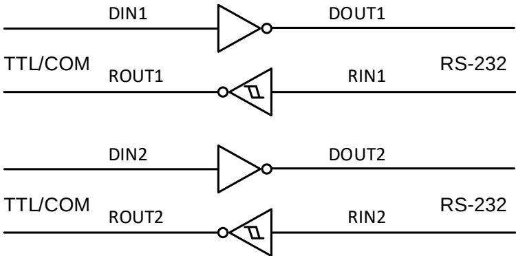
图 9-1 驱动器和接收器逻辑框图
