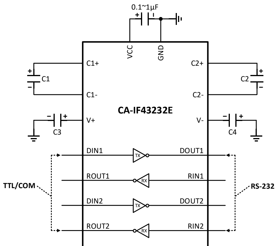
图 10-1 典型应用原理图
