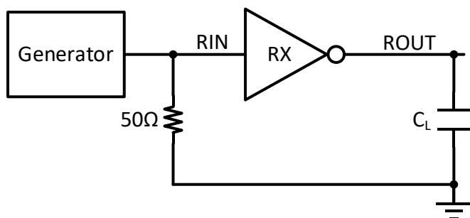
图 8-3 接收器传播延迟时间
