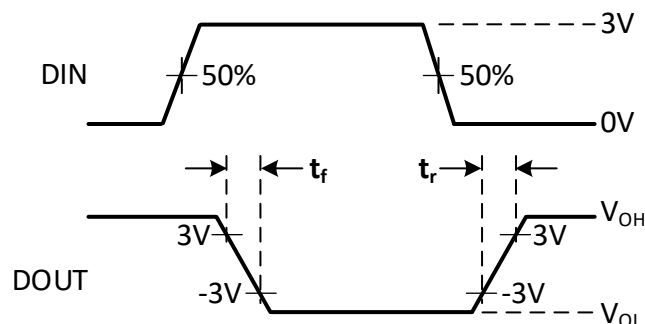
图 8-2 驱动器输出上升/下降时间
