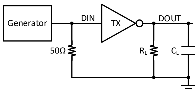
图 8-2 驱动器输出上升/下降时间
