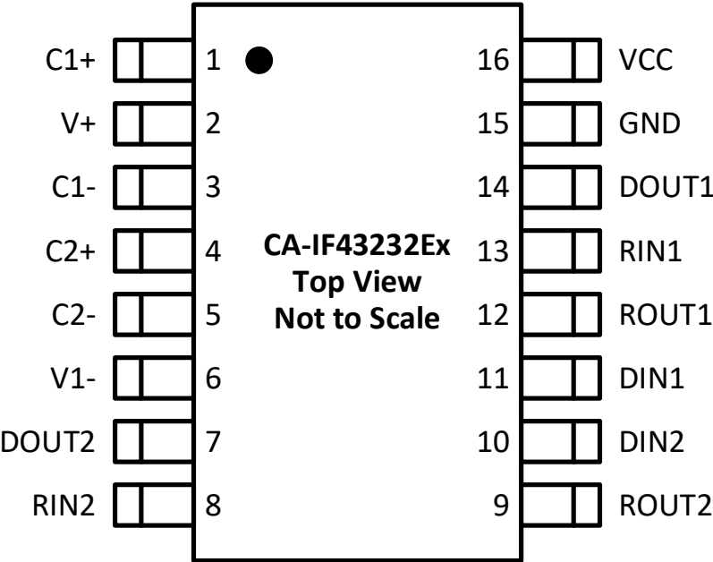
图 6-1 引脚分布图
