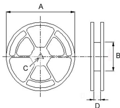
Reel Dimensions
