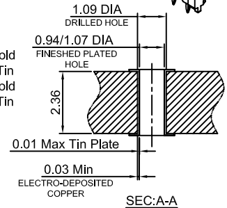
SEC:A-A
