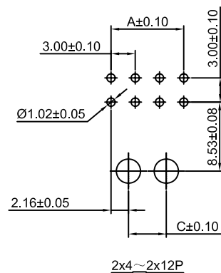
P.C.B LAYOUT
