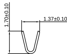
SEC:A-A
