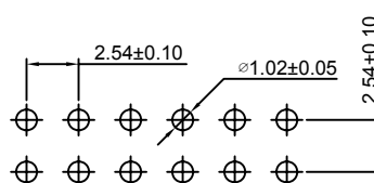
P.C.B LAYOUT
