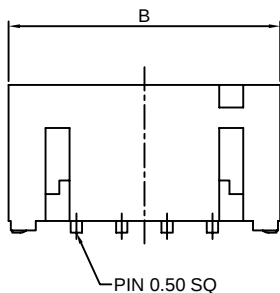
PIN 0.50 SQ
