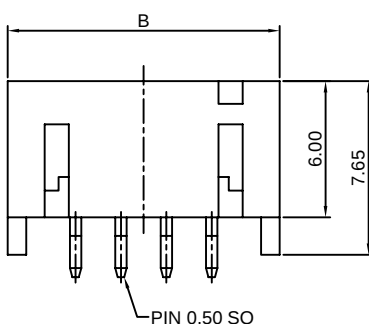
PIN 0.50 SQ
